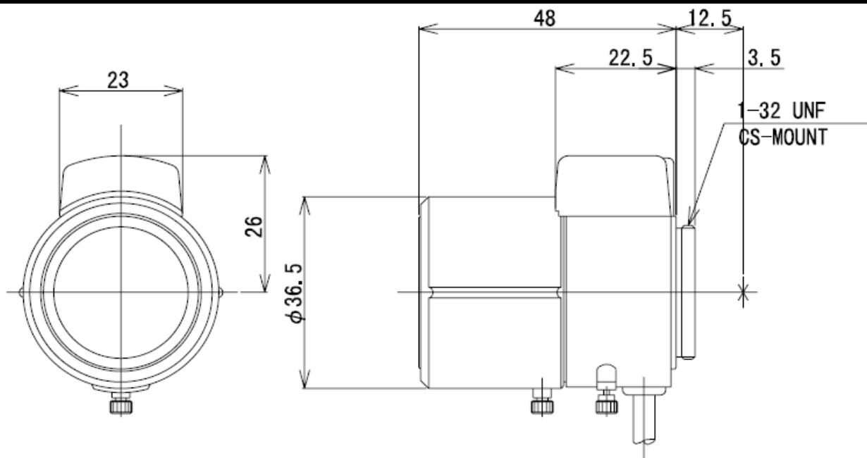
LMVZ41M ( P-Iris )
